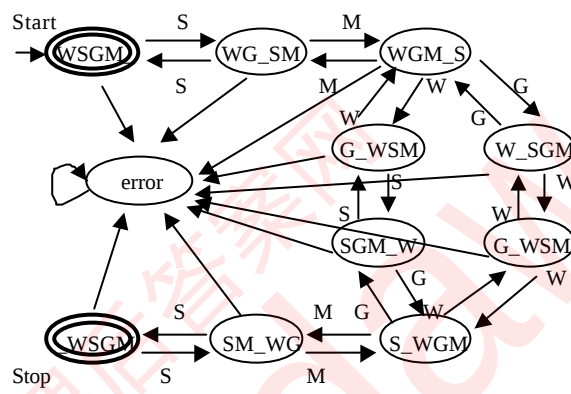
图 5.1 人带狼羊草过河的有限状态自动机
