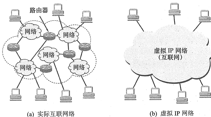
图 4.1 IP 网的概念
