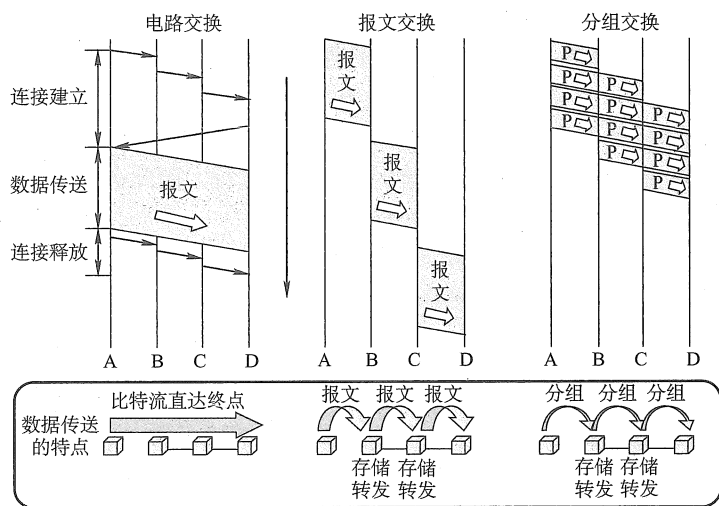
图 2.4 三种数据交换方式的比较
