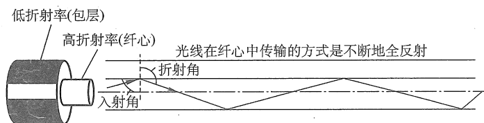
图 2.9 光波在纤心中的传播
