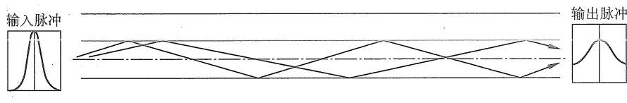
图 2.10 多模光纤
