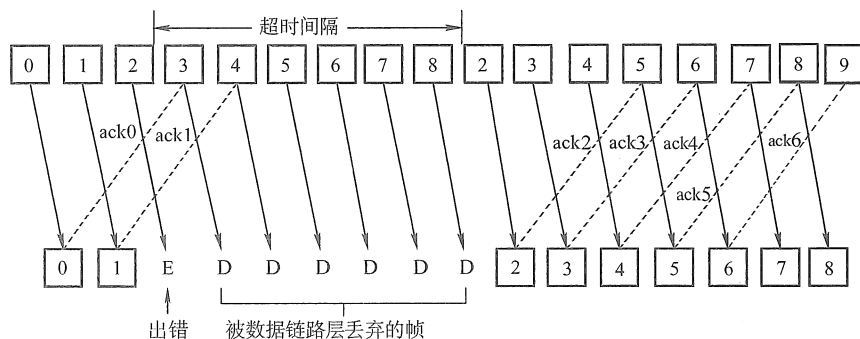
图 3.10 GBN 协议的工作原理:对出错数据帧的处理
