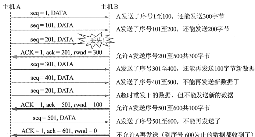
图 5.10 利用可变窗口进行流量控制举例
