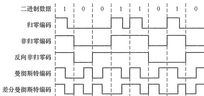
图 2.2 三种常用的数字数据编码方式
