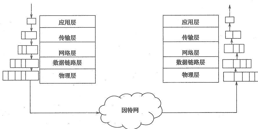
图 1.14 通信协议栈的通信用过程示例
