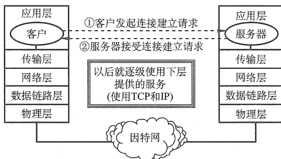
图 1.13 网络的五层协议体系结构模型
