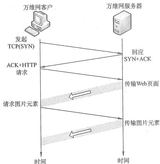
图 6.13 使用持久连接 (非流水线)
