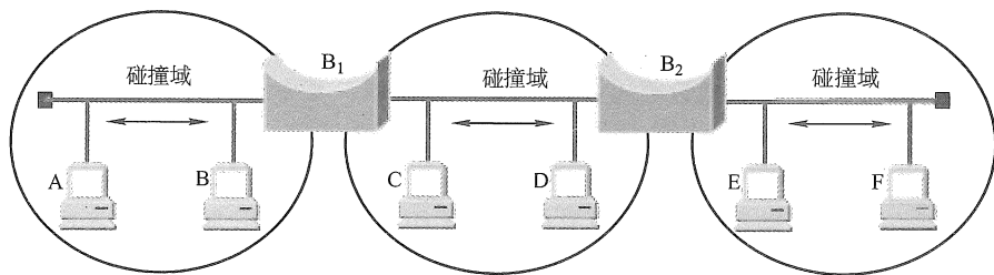
图 3.32 网桥使各网段成为隔离开的碰撞域
