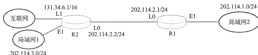
图 4.13 一个简单的网络拓扑
