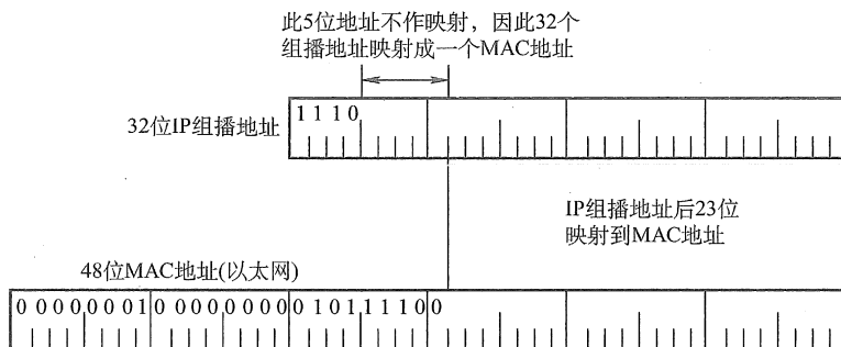
图 4.11 D 类 IP 地址与以太网组播地址的映射关系
