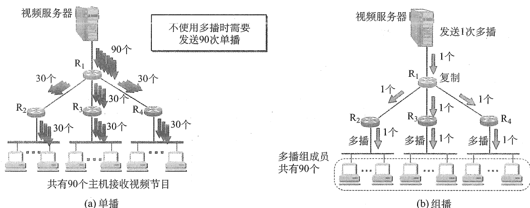
图 4.10 单播与组播的比较
