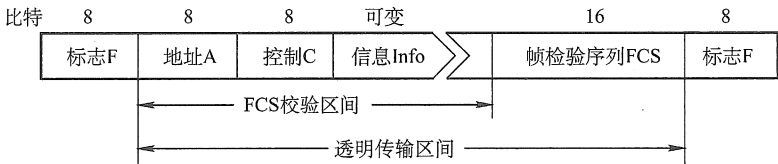
图 3.31 HDLC 的帧格式
