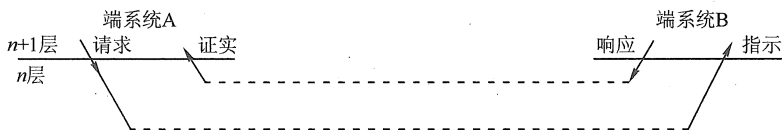
图 1.6 4 类原语的关系
