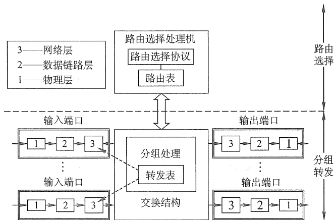
图 4.12 路由器体系结构
