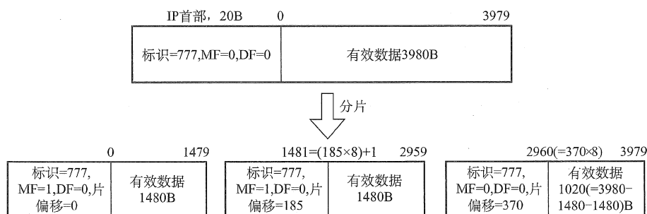
图 4.4 IP 分片的例子
