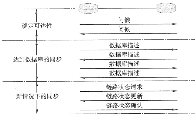
图 4.8 OSPF 的基本操作
