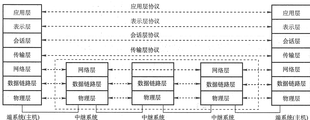
图 1.8 OSI 的层次结构
