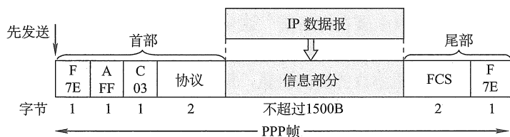
图 3.29 PPP 帧的格式
