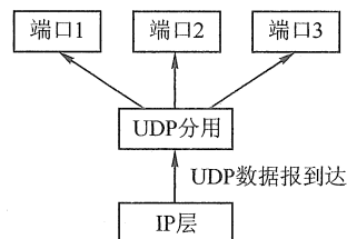
图 5.3 UDP 基于端口的分用
