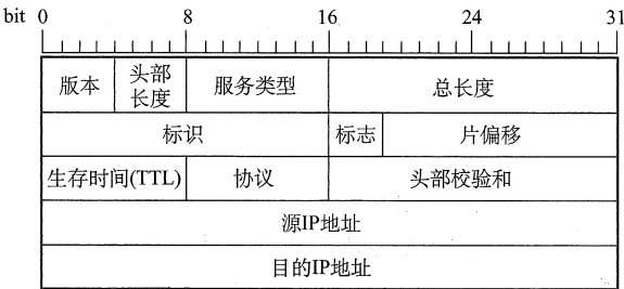
图 1 IP 分组头结构
