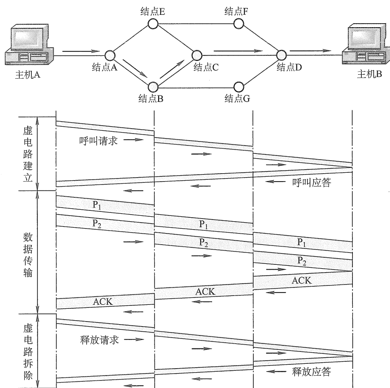
图 2.6 虚电路方式的工作原理
