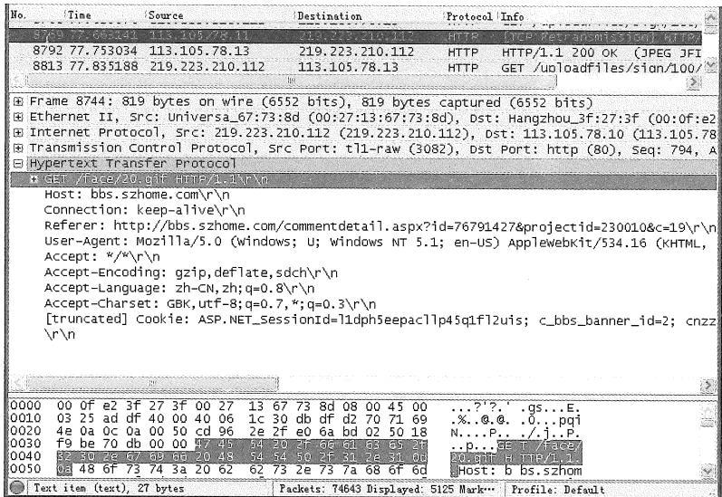
图 6.15 使用 Wireshark 捕获的 HTTP 请求报文的示例
