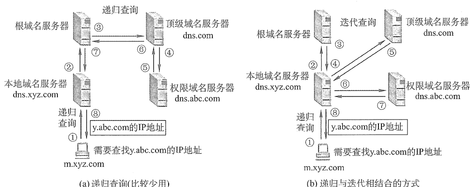
图 6.6 两种域名解析方式工作原理
