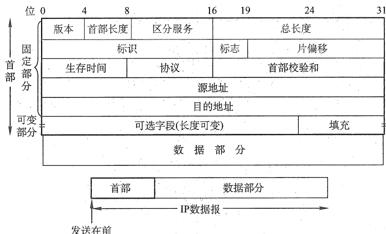
图 4.3 IP 数据报的格式
