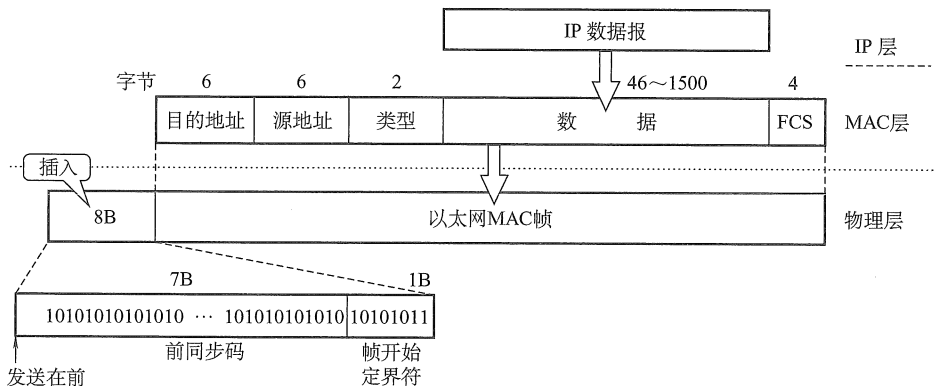
图 3.24 以太网 V2 标准的 MAC 帧格式
