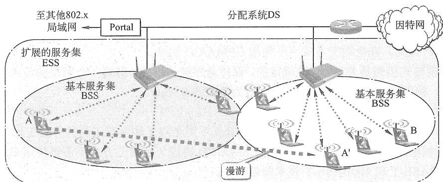
图 3.25 基本服务集和扩展服务集
