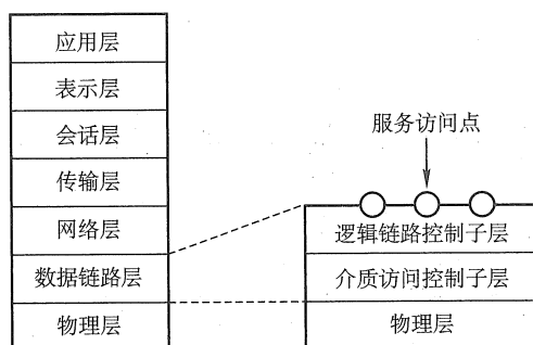
图 2.23 IEEE 802 协议层与 OSI 模型比较
