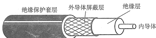
图 2.8 同轴电缆的结构
