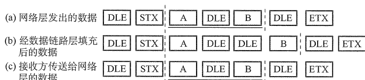
图 3.4 字符填充法
