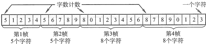
图 3.3 字符计数法
